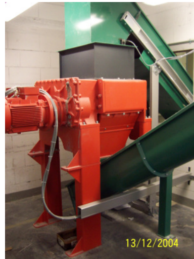
Vorzerkleinerung
